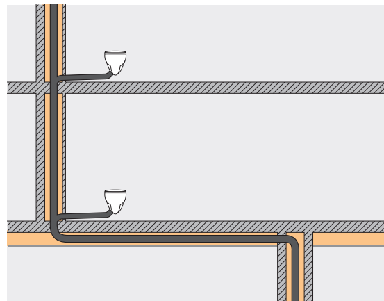
Aangezien SuperTube-afvoersystemen geen verboden zones hebben voor aansluitingen, zijn extra verluchtungsleidingen niet nodig. Horizontale delen kunnen zonder helling geplaatst worden.
