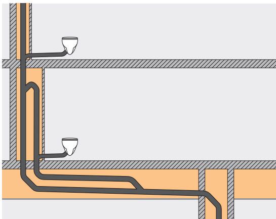
Conventioneel afvoersysteem: standleiding met verluchtungsleiding en helling in de horizontale delen
